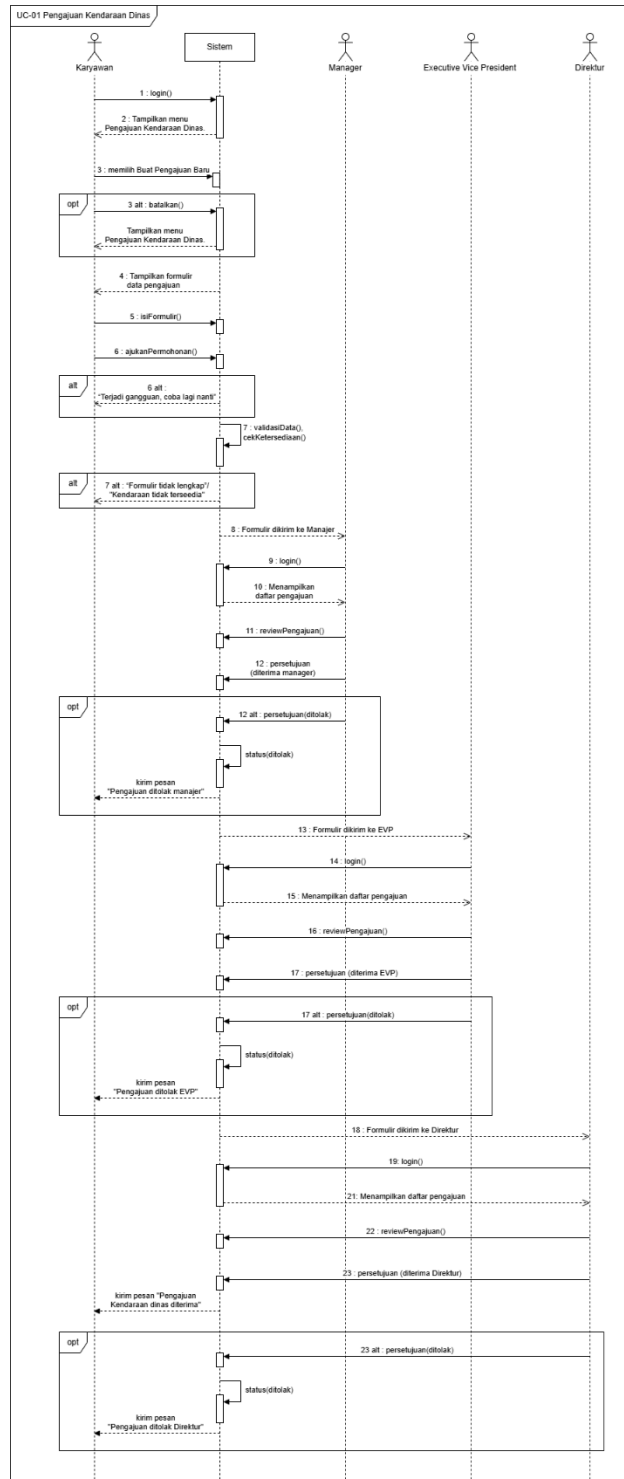
Gambar 3. 27 Sequence Diagram Pengajuan Kendaraan Dinas
